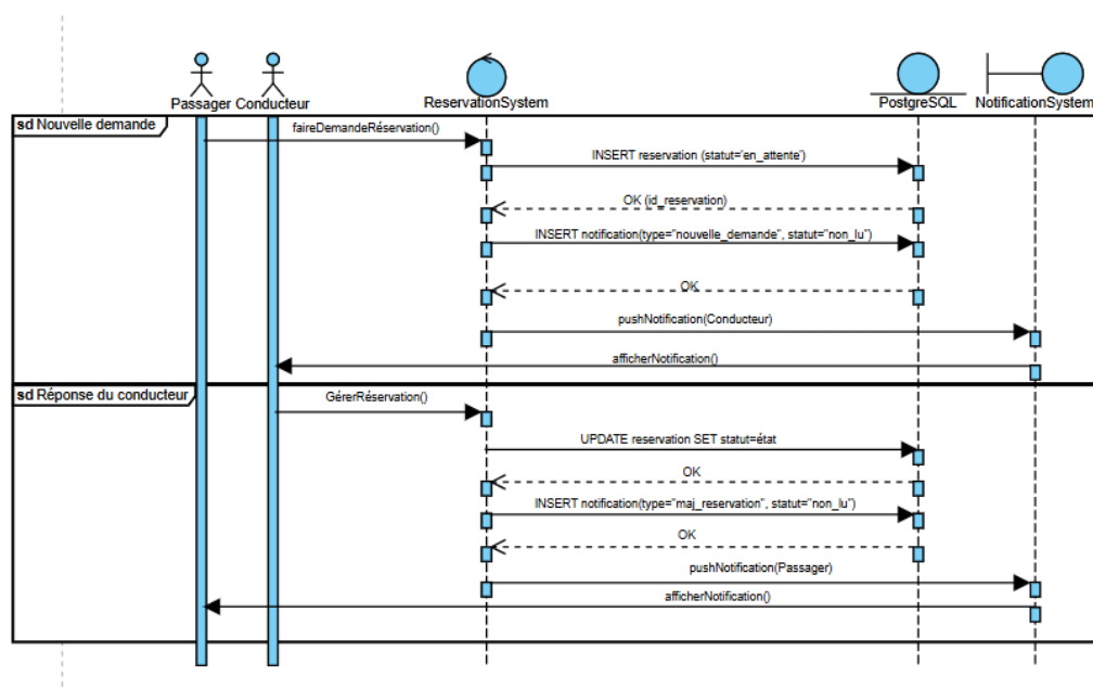
Diagramme de séquence qui illustre le mécanisme d'envoi et de réception des notifications dans le système
